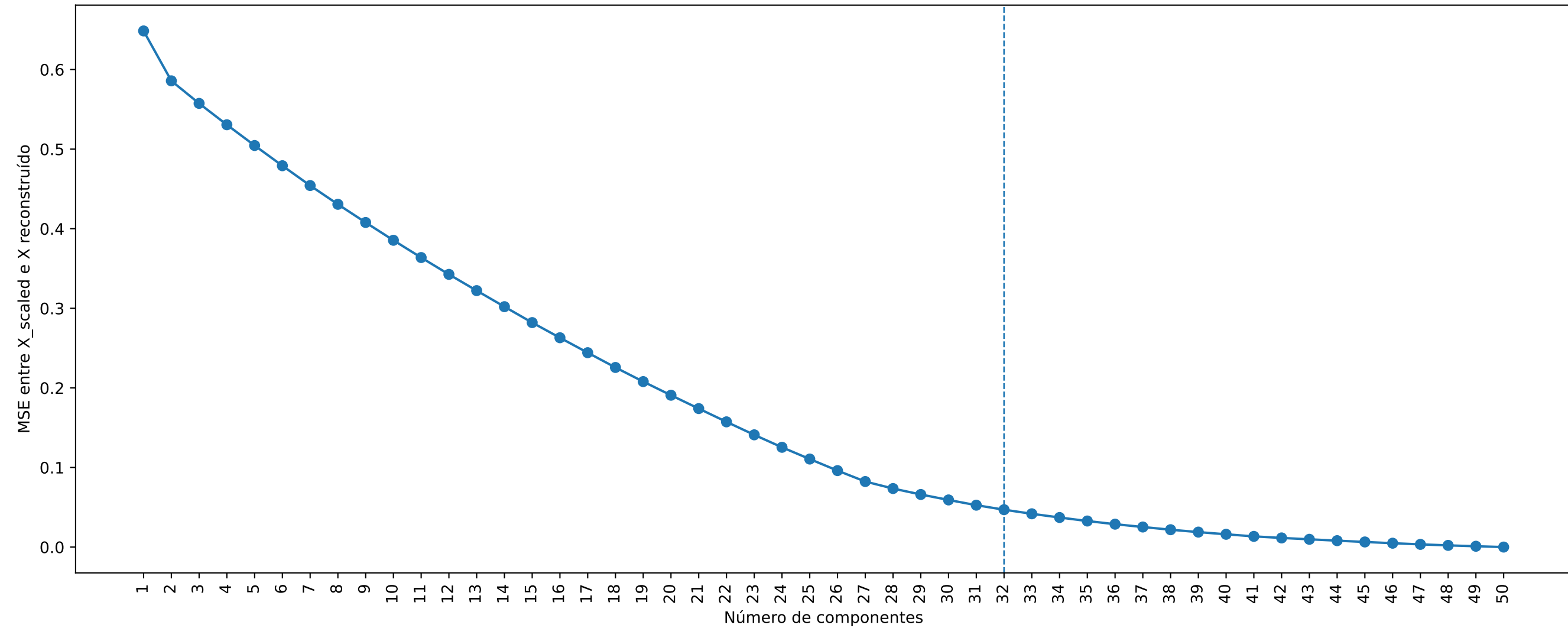
Erro de reconstrução por número de componentes
